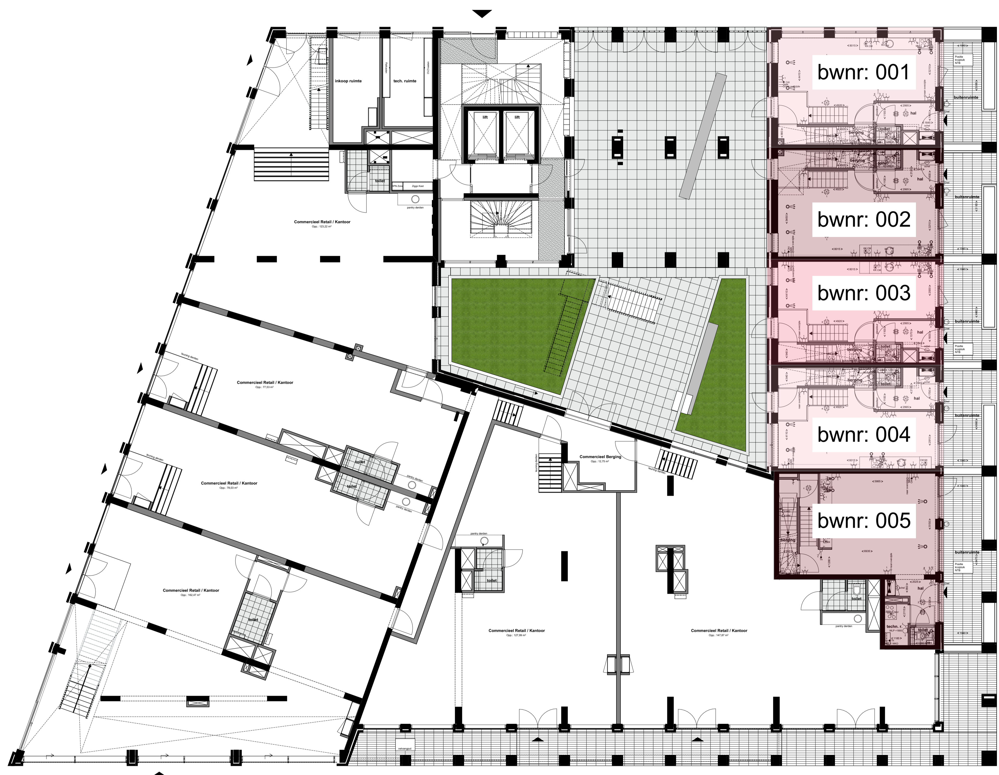
begane grond 1:100
