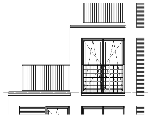
Zuid-Gevel 1:100
