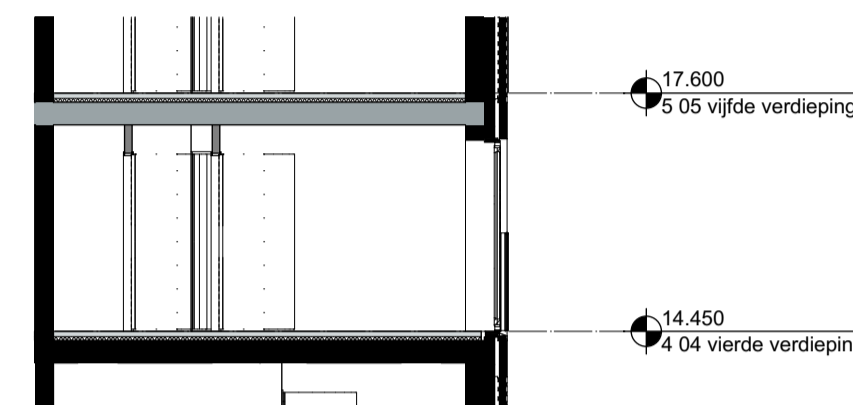
Doorsnede 1:100
